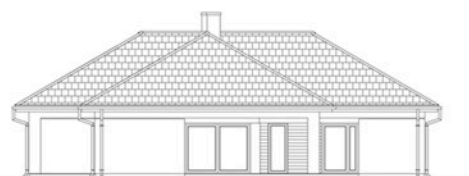
elewacja boczna/ogrodowa
