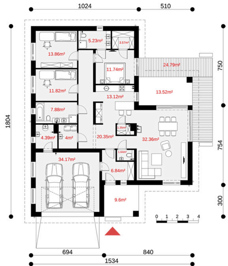
rzut parteru
