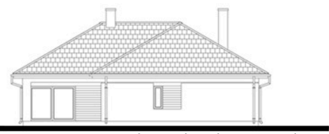
elewacja tylna/ogrodowa
